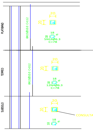
PILARES COM SEÇÃO 20X20 1:50
