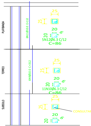
PILARES COM SEÇÃO 25X25 1:50
