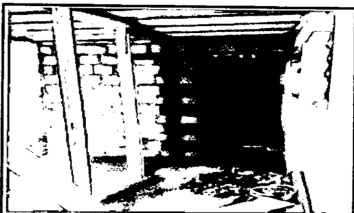
FOTO 01 - EXECUÇÃO DA ALVENARIA DE VEDAÇÃO DE BLOCOS CERÂMICOS FURADOS NA HORIZONTAL DE 9X19X19CM (ESPESSURA 9CM) DE PAREDES COM ÁREA LÍQUIDA MAIOR OU IGUAL A 6M² COM VÃOS E ARGAMASSA DE ASSENTAMENTO
