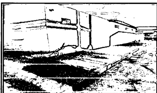
FOTO 20 - EXECUÇÃO DE PASSEIO (CALÇADA) OU PISO DE CONCRETO COM CONCRETO MOLDADO IN LOCO, FEITO EM OBRA, ACABAMENTO CONVENCIONAL, NÃO ARMADO. AF_07/2016
