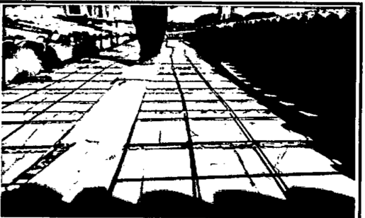
FOTO 05 - EXECUÇÃO DA LAJE PRÉ-FABRICADA TRELIÇADA PARA PISO OU COBERTURA, INTEREIXO 38CM, H=12CM, EL. ENCHIMENTO EM EPS H=8CM, INCLUSIVE ESCORAMENTO EM MADEIRA E CAPEAMENTO 4CM
